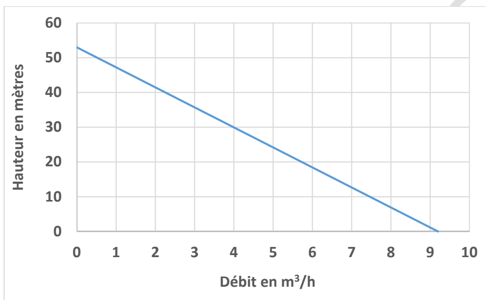
Figure 2 : Débit de la pompe en fonction de la hauteur de pompage
