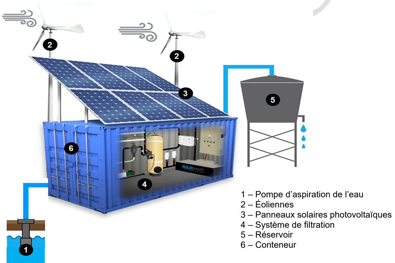
Figure 1 : schéma descriptif du système
