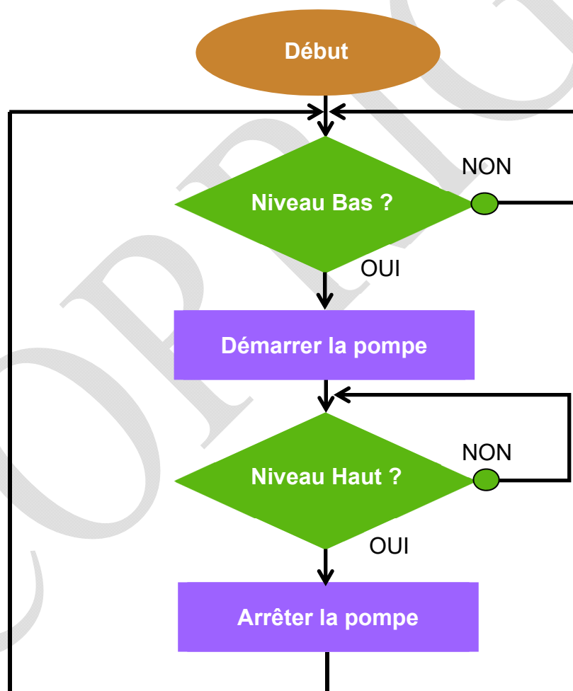
Figure 4 : algorithme du fonctionnement de la pompe
